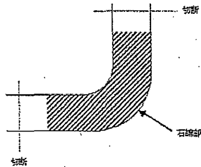
図 配管エルボの本例
