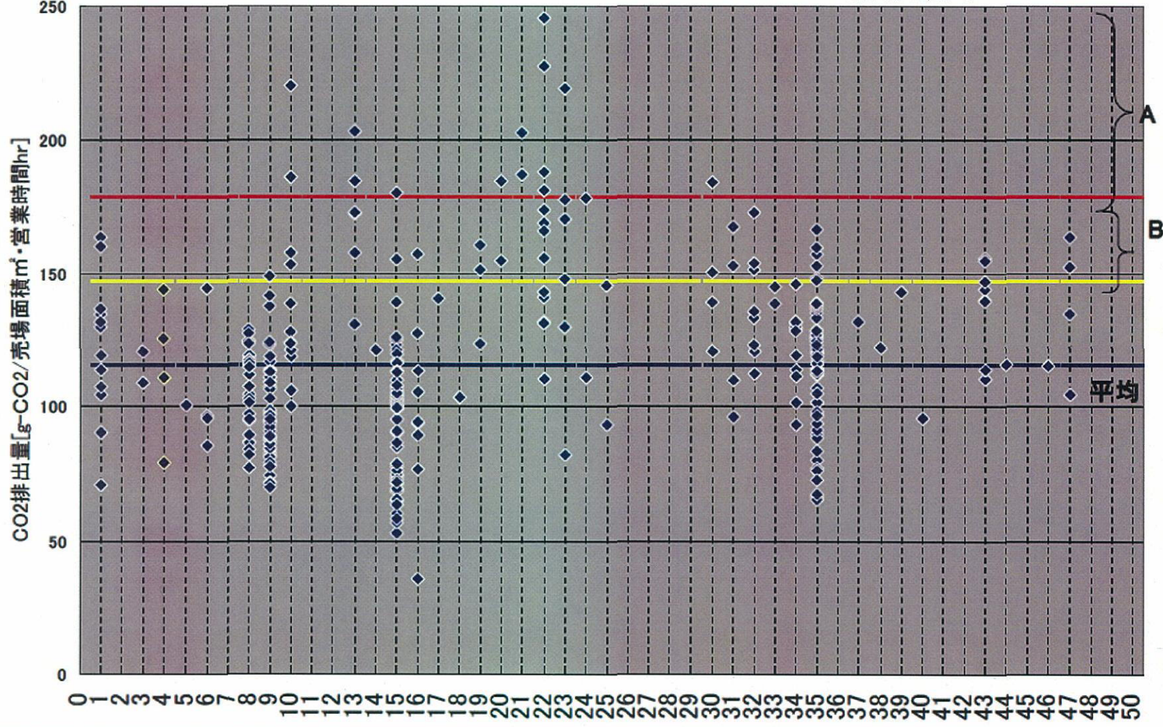
売場面積別CO2排出量原単位(売場面積・営業時間) 200坪未満
