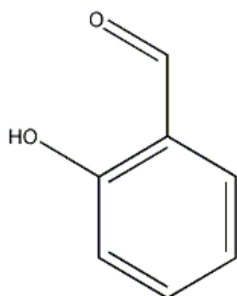
構造式
