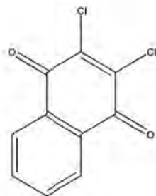
構造式
