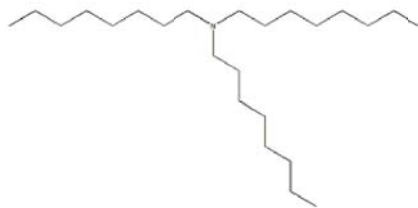
構造式
