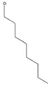
構造式
