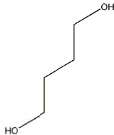
構造式
