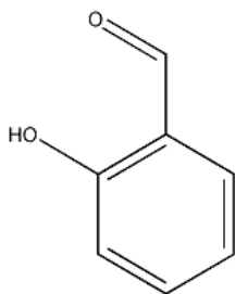
構造式
