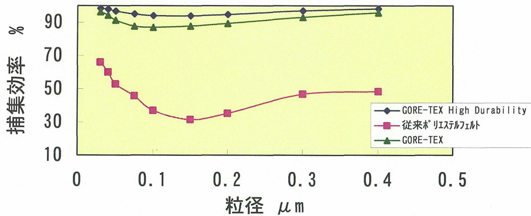
捕集効率vs. 粒径 (550g/m 2 PEフェルト 濾過速度3m/min)
