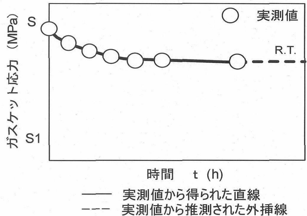
図2 ガスケット応力緩和曲線
