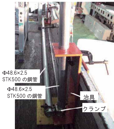
図 3-17 支柱下端を鋼管で連結した状態
