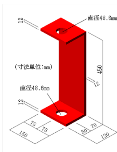
図 3-18 治具の寸法
