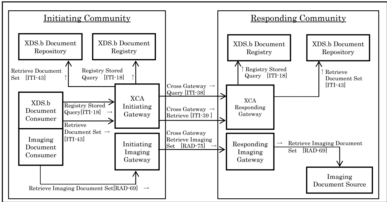
図 15.1 Cross-Community Access for Imaging(XCA-I)のアクタおよびトランザクション
