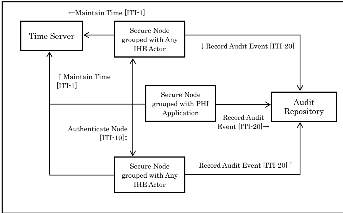
図 17.1 Audit Trail and Node Authentication (ATNA)のアクタおよびトランザクション
