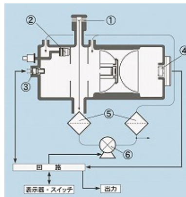
図-22 粉じん相対濃度計の構造の例
