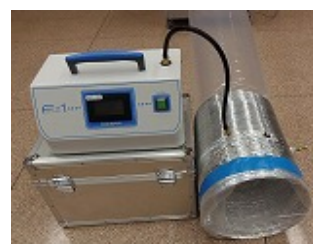
繊維状粒子自動測定機
