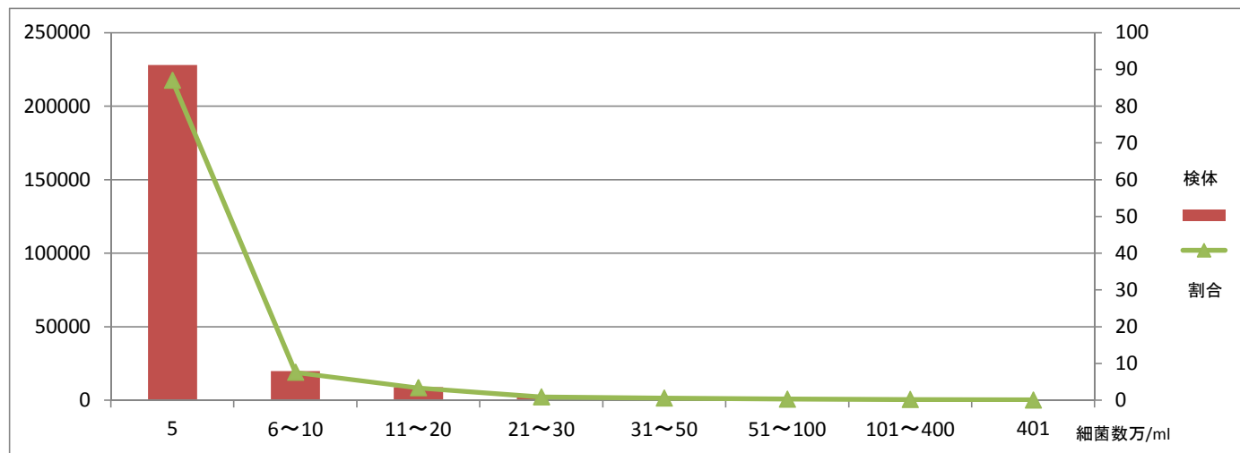
○バルク乳における細菌数の分布図(平成25年度)
