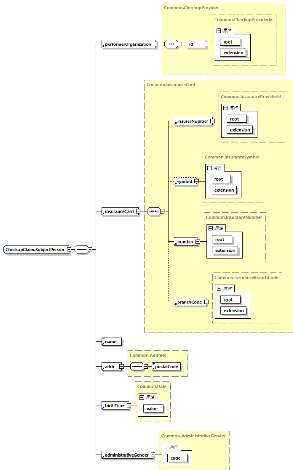
図 3 XML スキーマの構造 (受診者情報)
