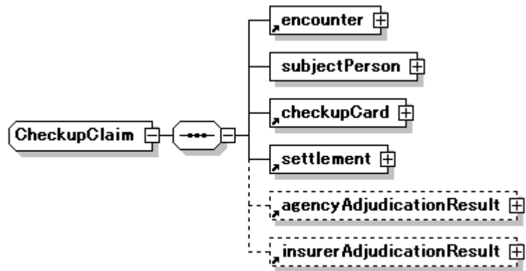
図 1 XML スキーマの構造 (全体構造)
