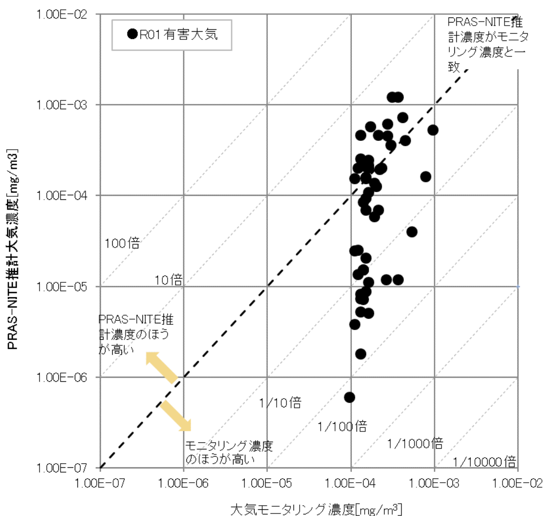
262 図 5 PRAS-NITE の推計大気濃度 (PRTR、令和元年度) と
