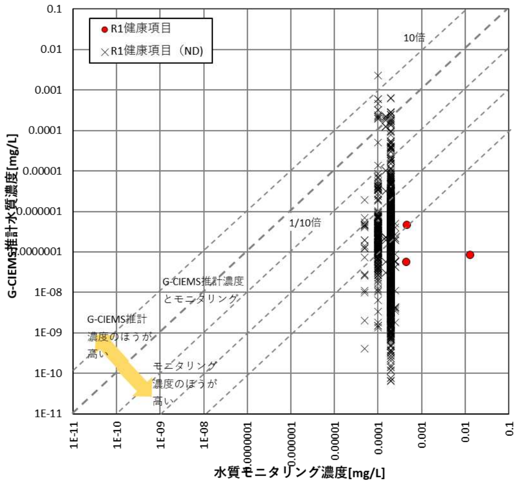
図 4 G-CIEMS の推計水質濃度 (PRTR、令和元年度) とモニタリング水質濃度 (健康項目 (令和元年度)) の比較 78
