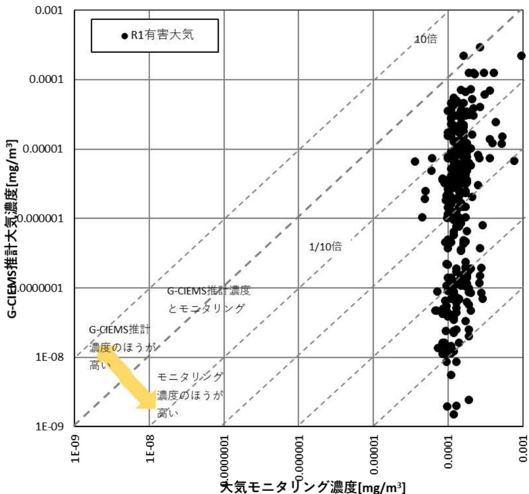
249 図 3 G-CIEMS の推計大気濃度 (PRTR、令和元年度) と
