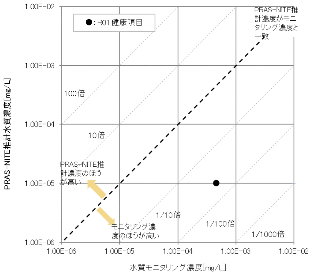
図 6 PRAS-NITE の推計水質濃度 (PRTR、令和元年度) とモニタリング水質濃度 (健康項目 (令和元年度)) の比較
