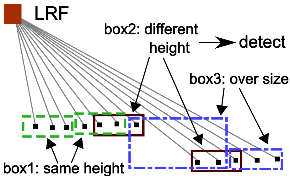
図 C-1-16 下り段差検知法
