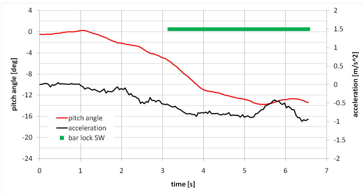
図 C-2-21 上り斜面走行実験 (8° の斜面, 制御あり)
