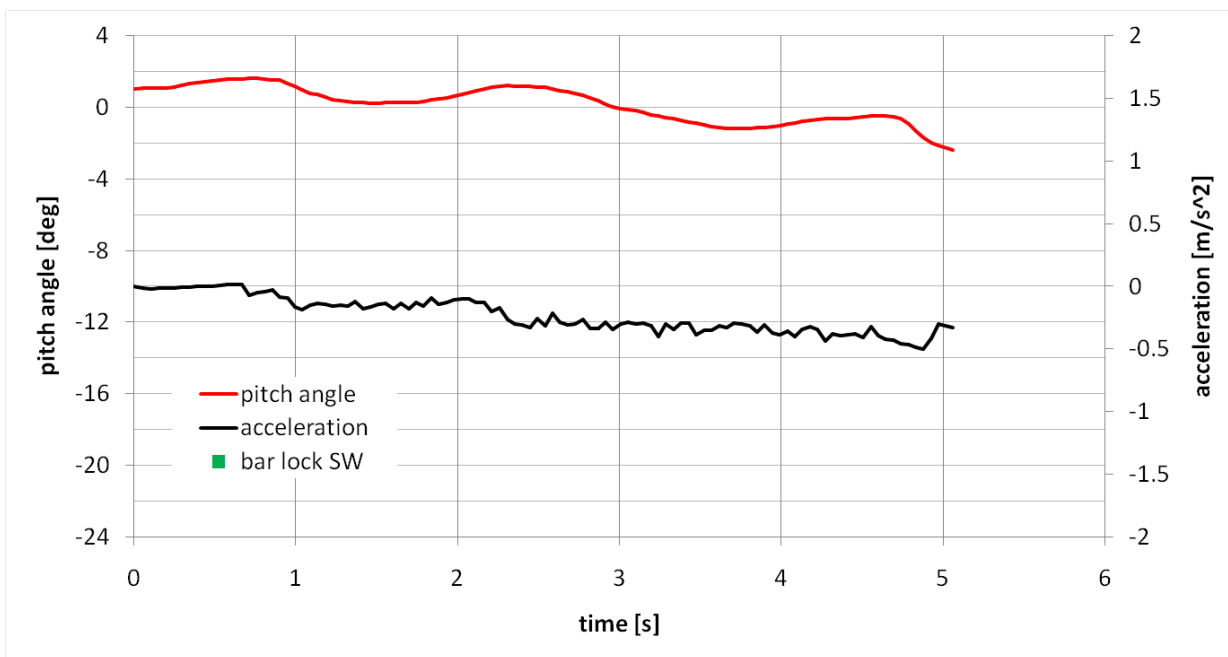
図 C-2-19 上り斜面走行実験 (6° の斜面, 制御あり)
