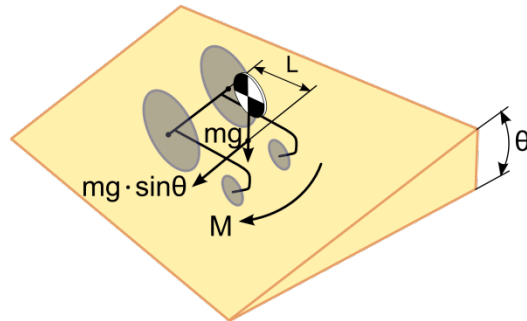
図 C-3-1 斜面横断時に車いすに作用する力
