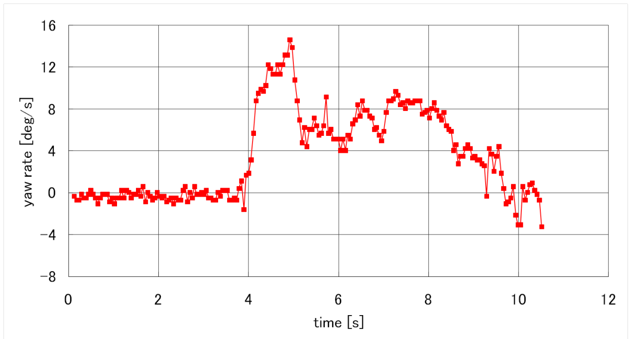
図 C-3-3 片流れ時のヨー角速度
