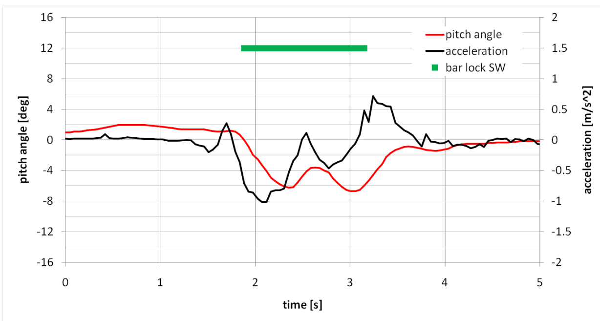
図 C-2-17 段差乗り越え実験（段差高さ 2.5cm, 助走なし, 制御あり）
