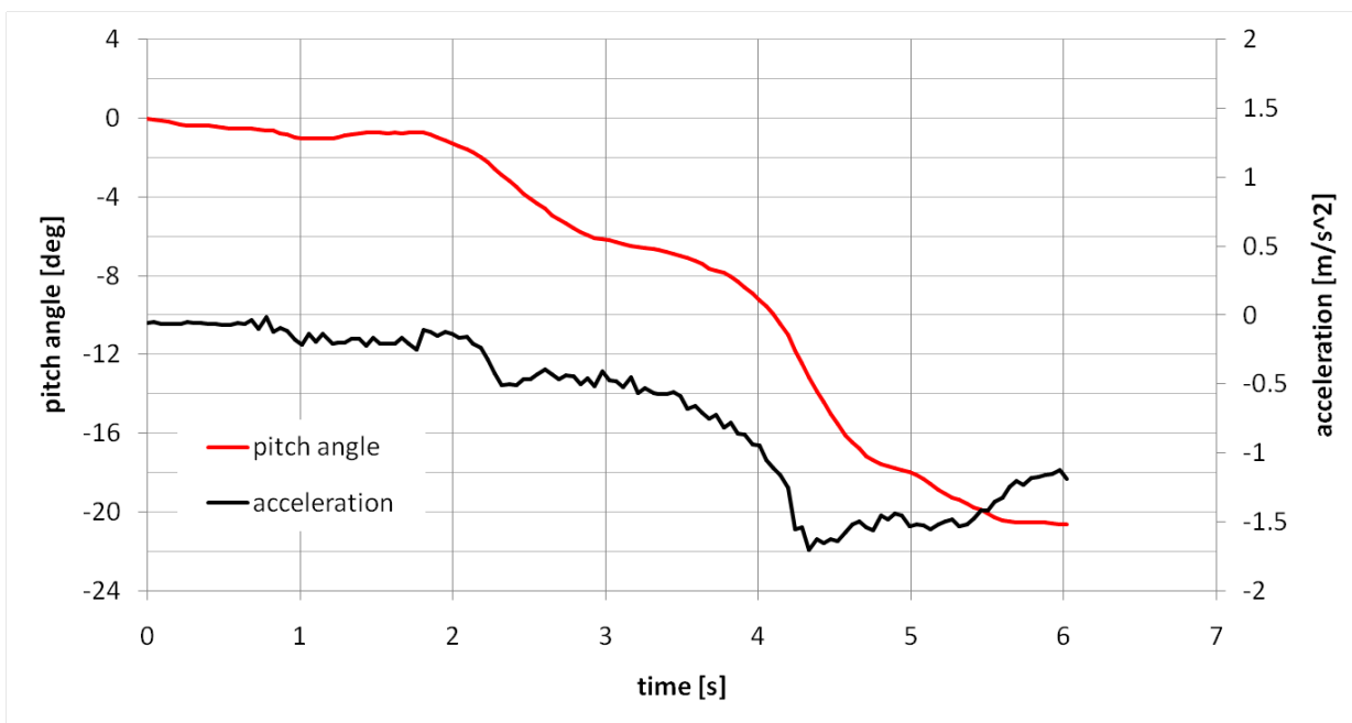
図 C-2-20 上り斜面走行実験 (8° の斜面, 制御なし)
