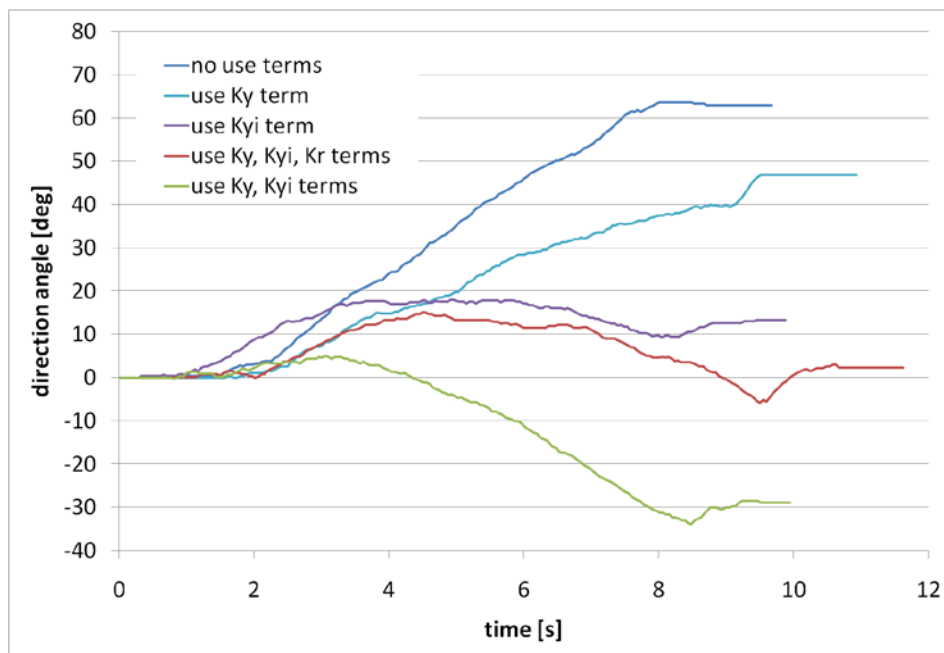
図 C-3-8 斜面横断実験
