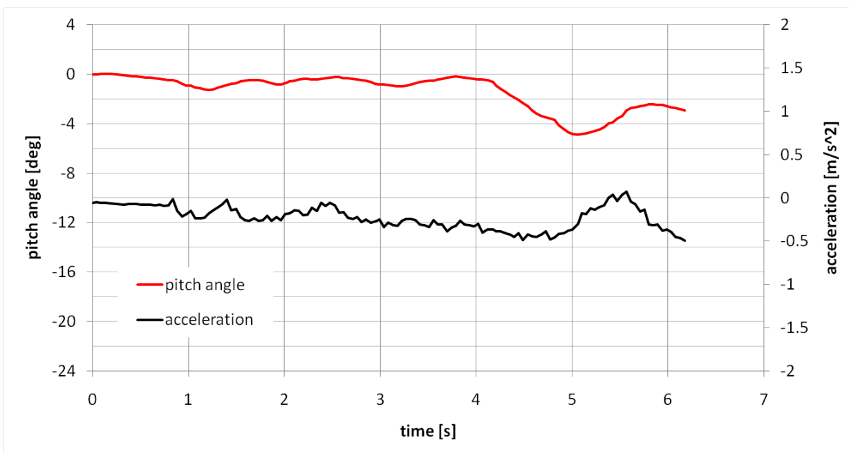
図 C-2-18 上り斜面走行実験 (6° の斜面, 制御なし)
