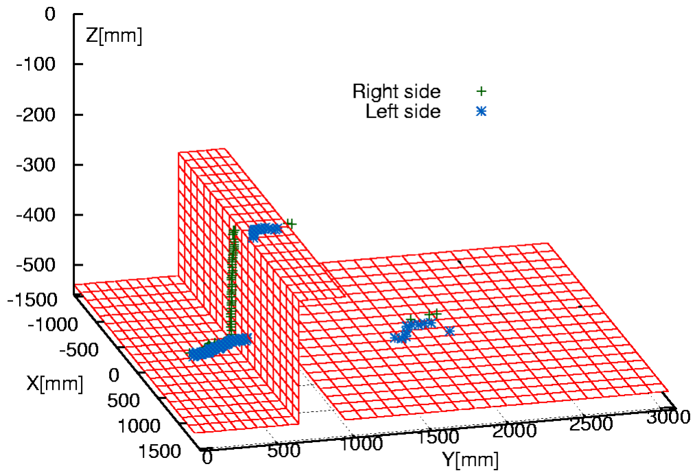
図 C-1-20 上り段差スキャン結果
