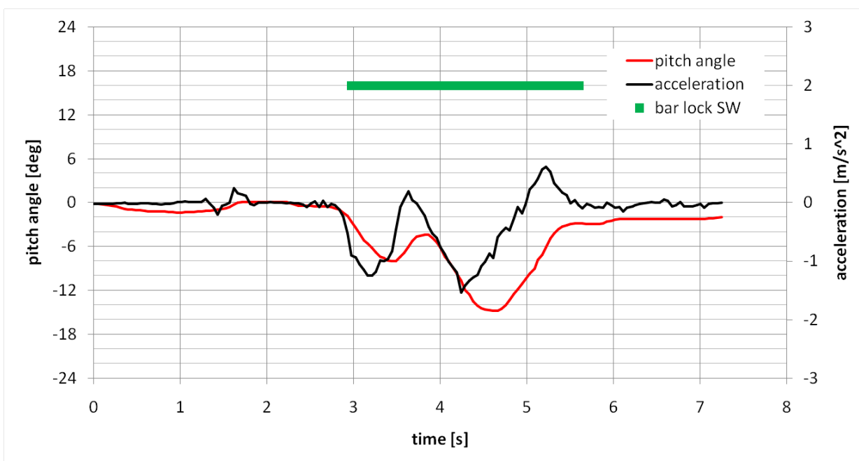
図 C-2-13 段差乗り越え実験（段差高さ 4.5cm, 助走なし, 制御あり）
