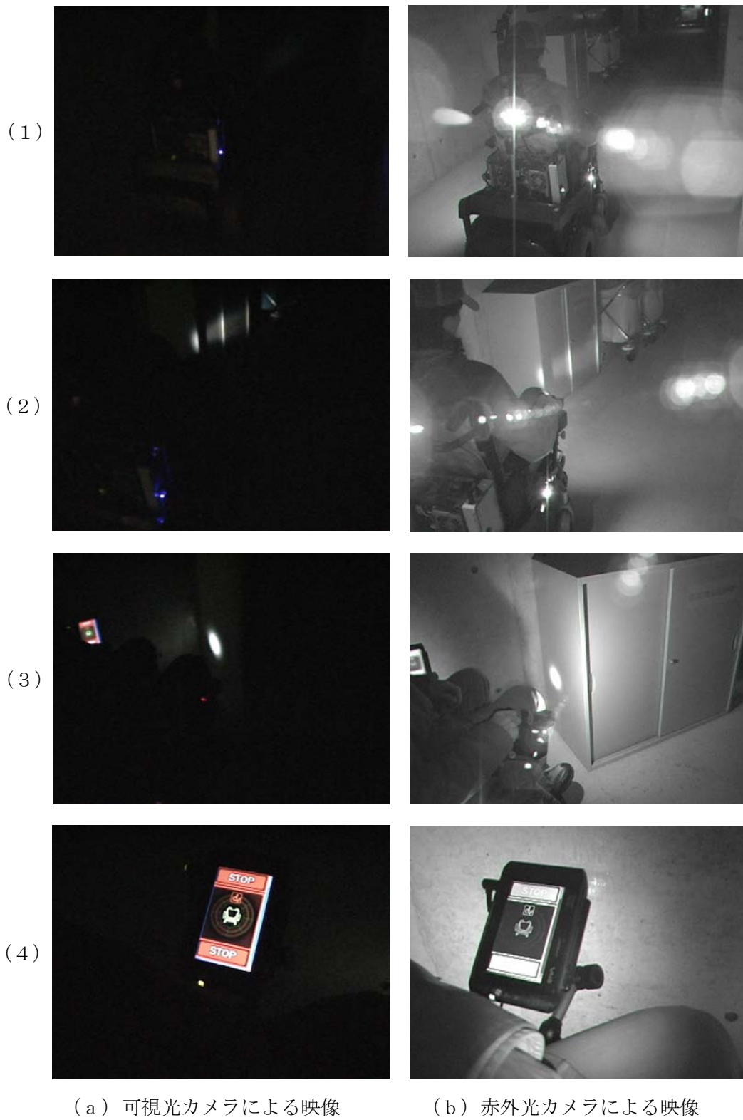
図 C-4-18 暗環境下での障害物の検知
