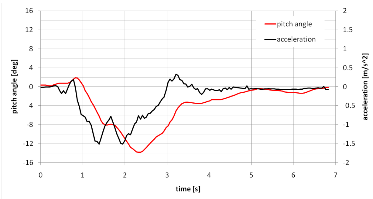
図 C-2-16 段差乗り越え実験（段差高さ 2.5cm, 助走なし, 制御なし）
