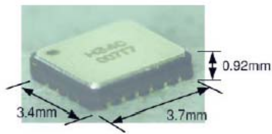
図 C-3-6 加速度センサ (H34C)
