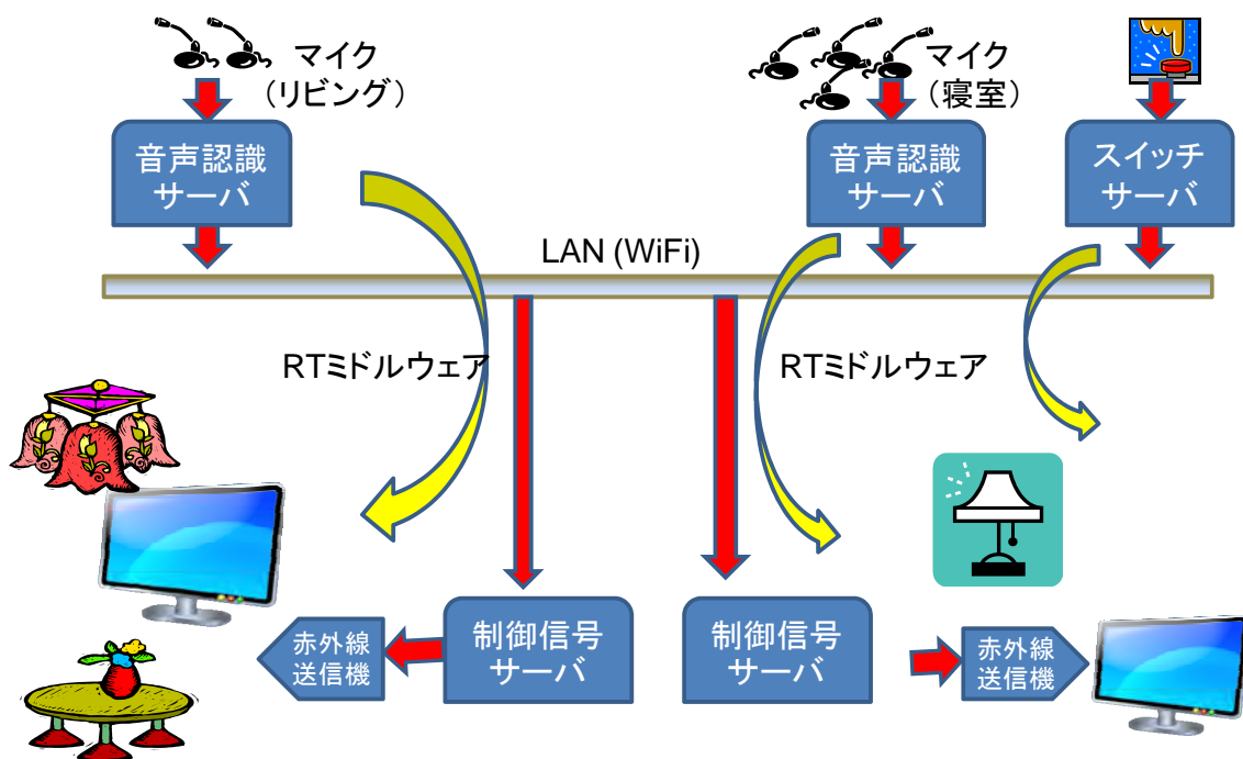
図 II-2-4 機器制御ネットワークの構成
