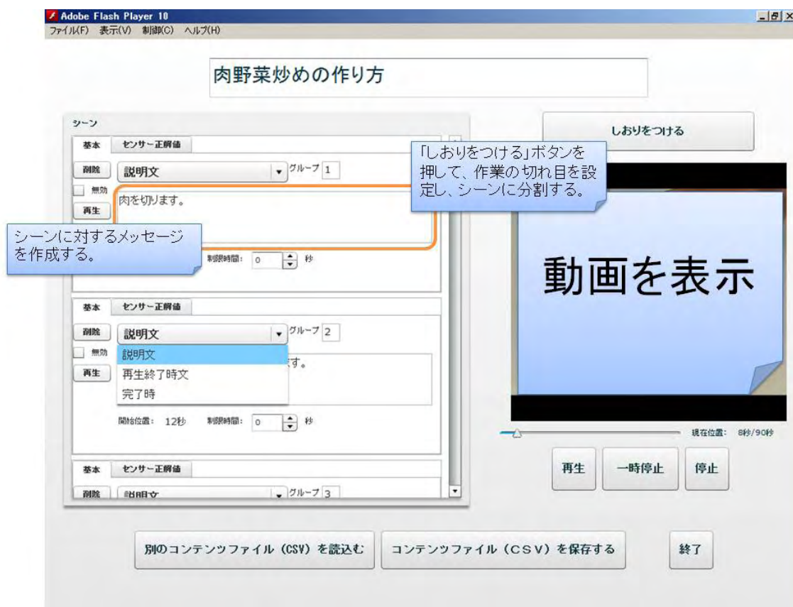
図 II-1-14 コンテンツ作成ツール（しおりの挿入とメッセージの作成）
